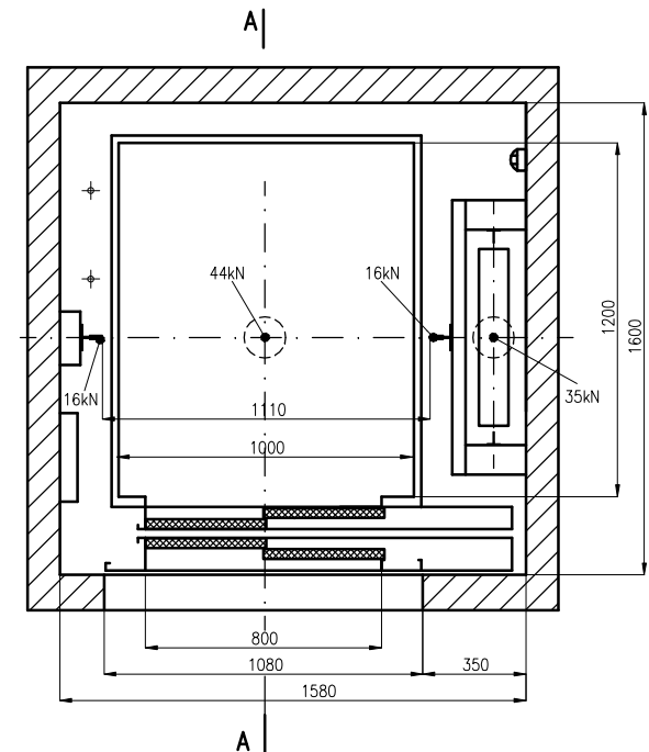
Rzut szybu B-B (1:20)
