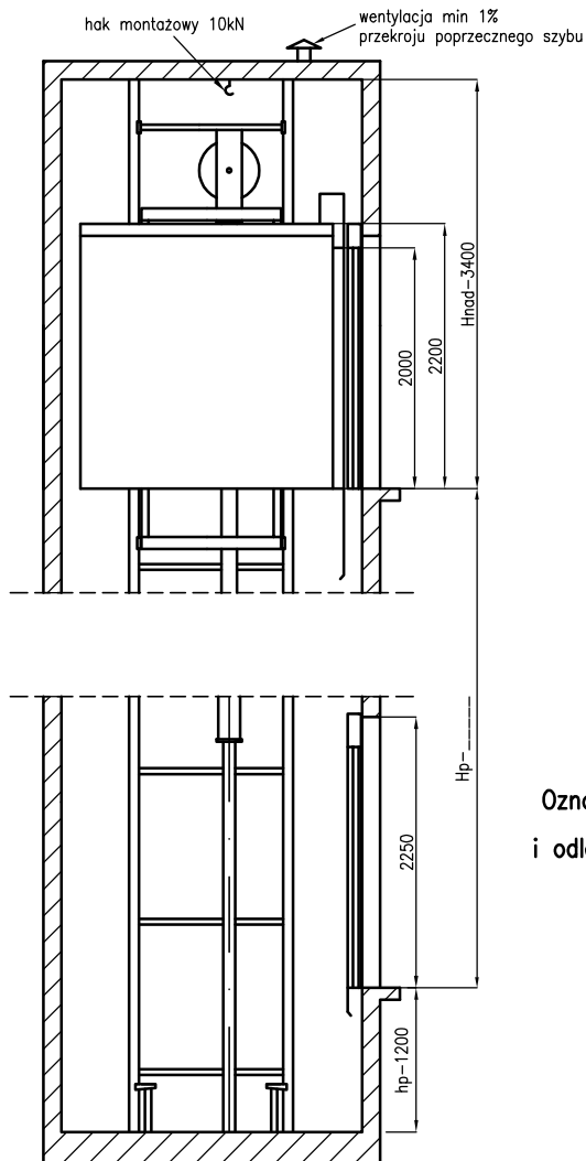
Przekrój pionowy szybu (1:50)
