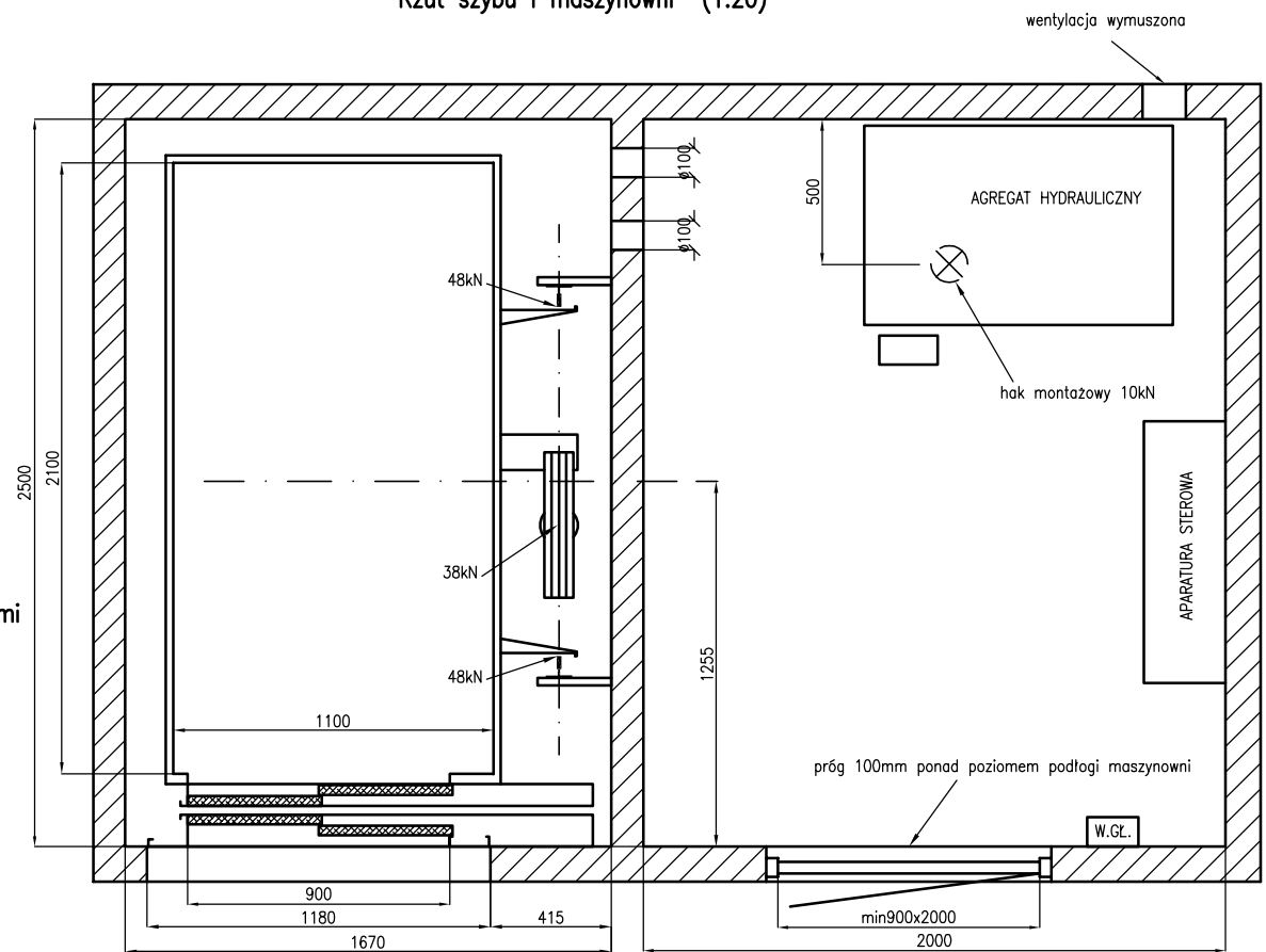
Rzut szybu i maszynowni (1:20)
