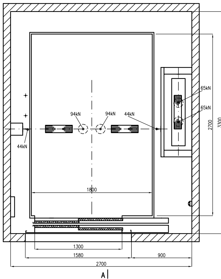
Rzut szybu B-B A|
