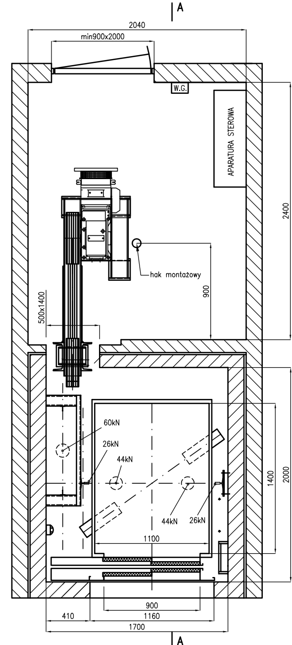
Rzut szybu i maszynowni C-C (1:25)
