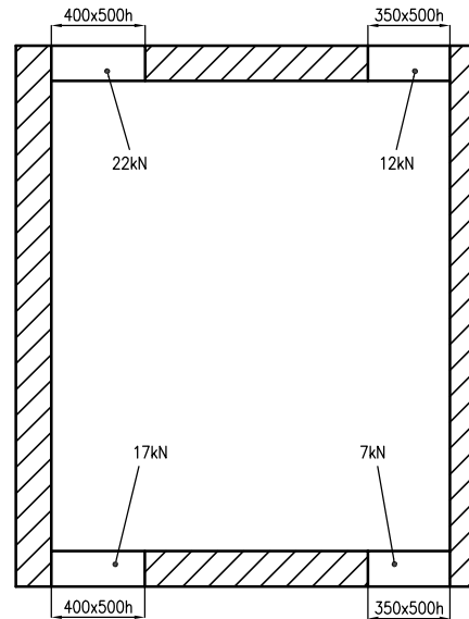
Plan otworów w nadszybiu B-B (1:25)
