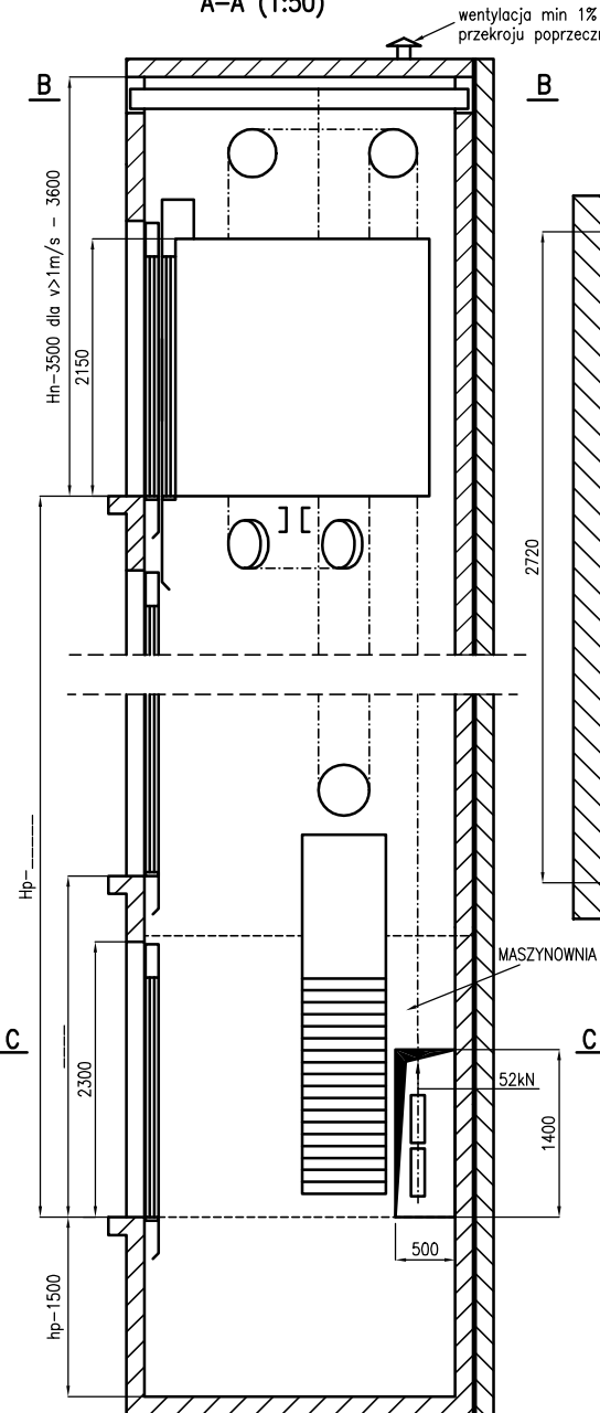
A-A (1:50)
