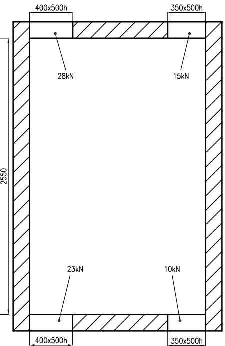
Plan otworów w nadszybiu B-B (1:25)
